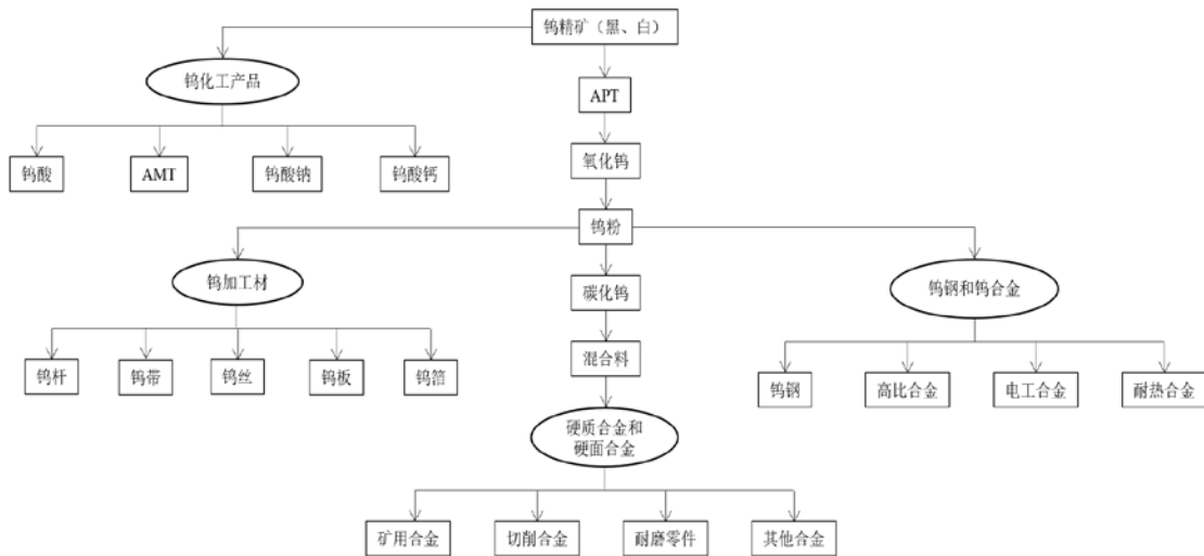
图 4-1 钨产业链图
